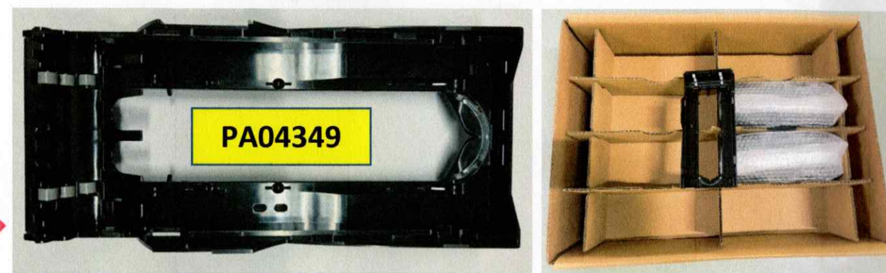
图一, PA04349 每箱 2 层, 每层 8 格, 每格放 2 个, 一个气泡袋装 2 个组件, 一箱装 32 个, 确认成品实物与要求一致后装进箱子。
